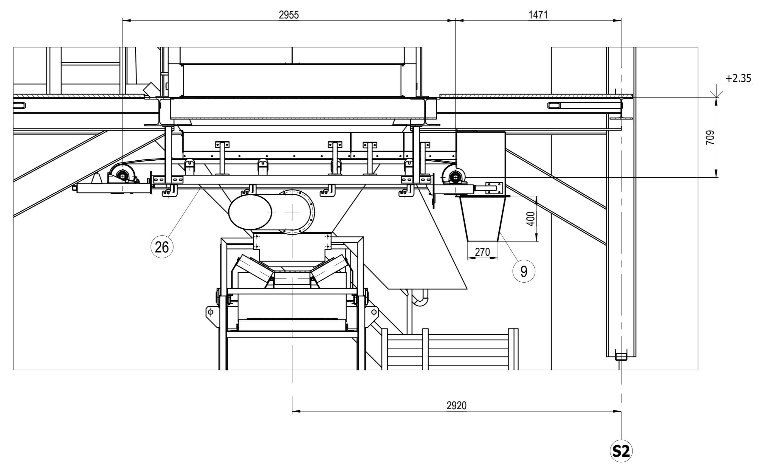
Д-Д (1:20)
