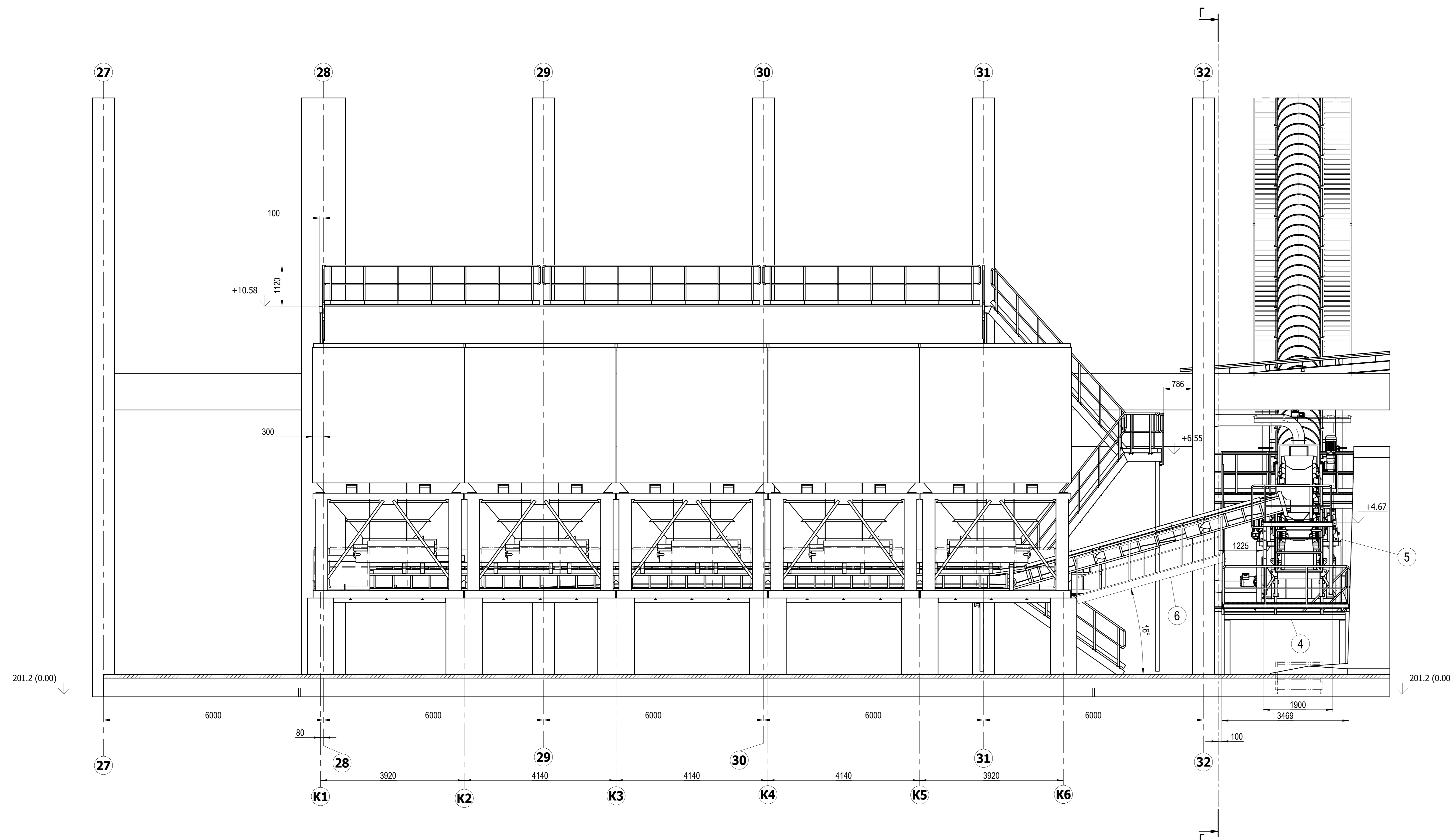
A-A (1:50)
